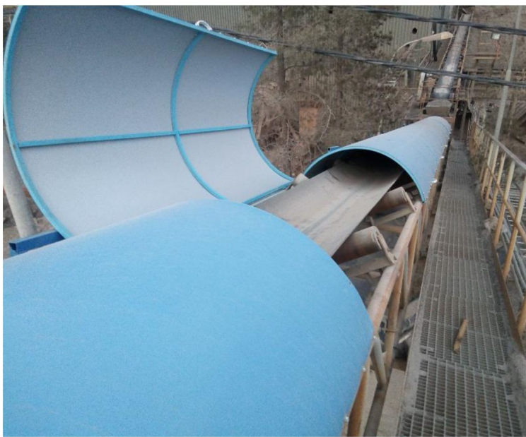
اجرای کامل خطوط انتقال مواد با پوشش
